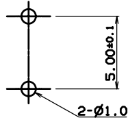
P.C.B DIMENSION
