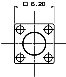
P.C.B DIMENSION
