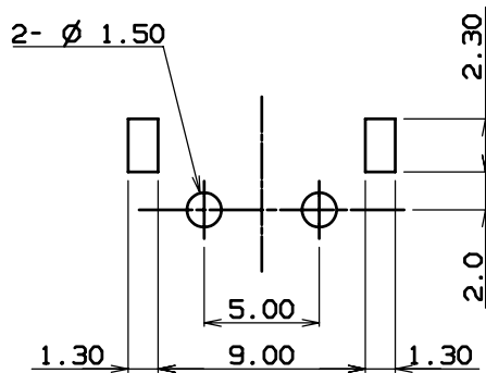
P.C.B DIMENSION
